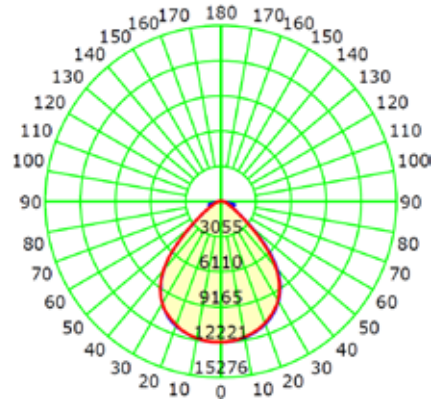
90°x90° (320W-HV)
