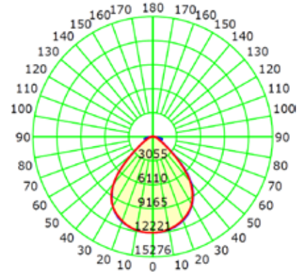
90°x90° (320W)
