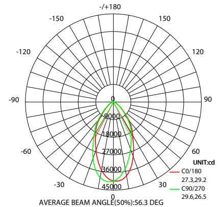
60°(300W-5000K)
