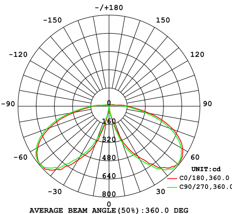
HL-BL-MW-MCCT-24W-CR (4000K)
