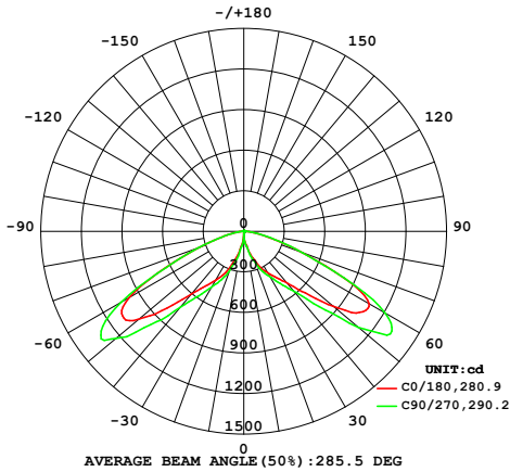
HL-BL-MW-MCCT-24W-DC (4000K)
